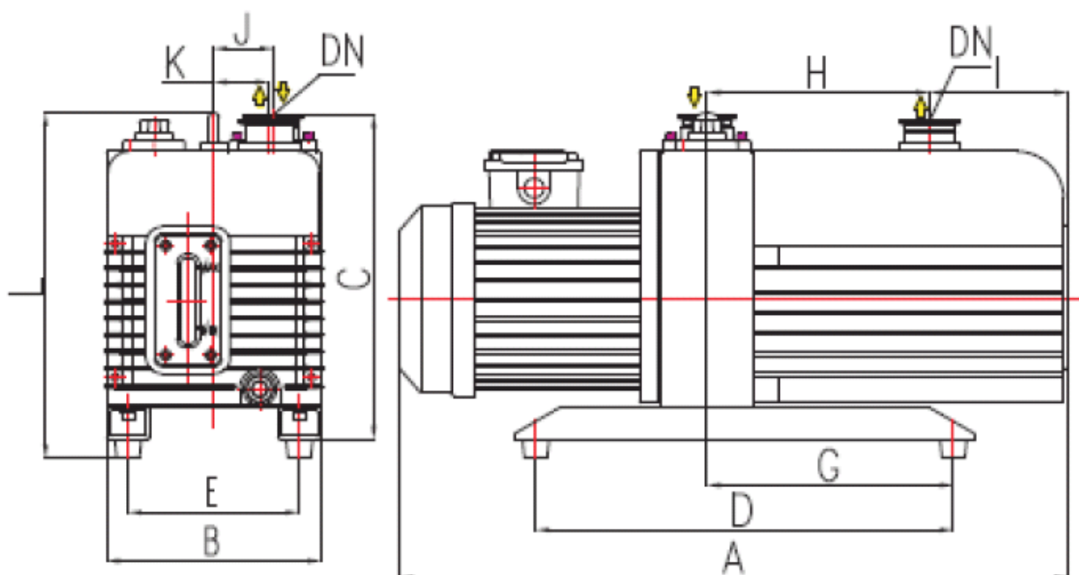
Габаритные размеры насоса серии VRD
